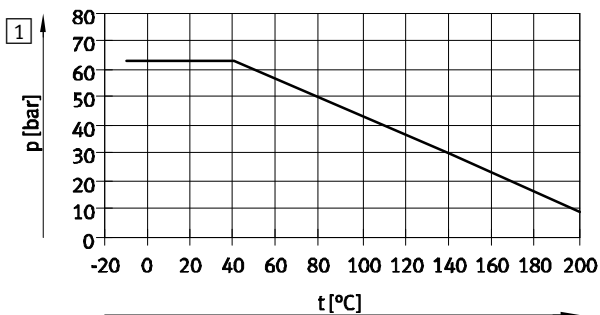
Fig. 5 Druck – Temperatur-Diagramm
