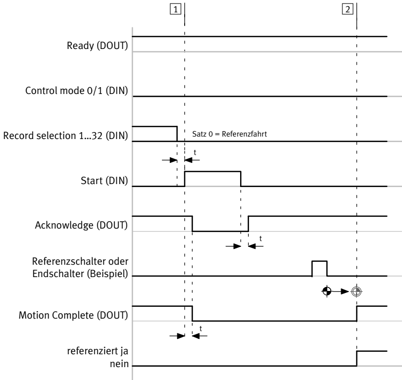
Fig. 2.23 Zeitdiagramm Modus 0; Referenzfahrt auf Referenzschalter oder Endschalterschalter
