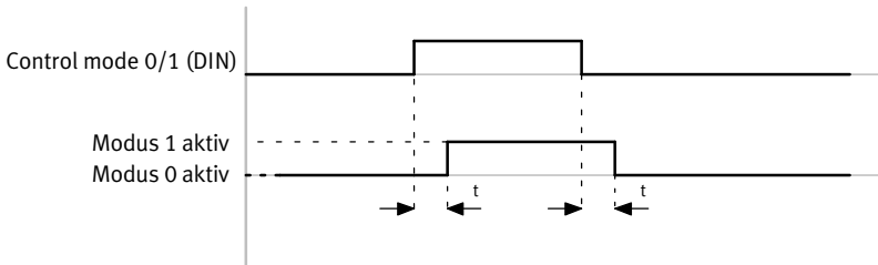
Fig. 2.20 Zeitdiagramm Modus der I/O-Schnittstelle einstellen
