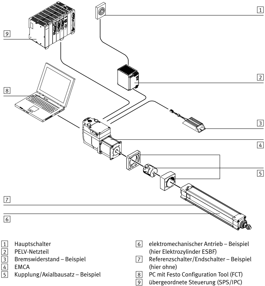
Fig. 2.2 Systemaufbau (Beispiel)
