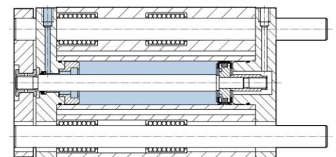
Fig.10: Geleidingseenheid
