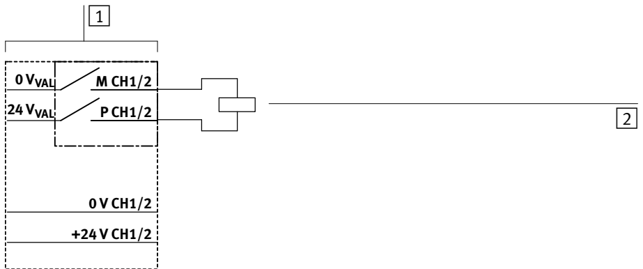
Bild 1/6: Sichere Abschaltung potenzialfreier Einzelverbraucher
