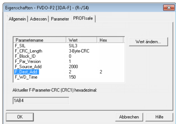
Bild 3/5: PROFIsafe-Parameter
