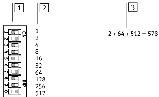
Bild 2/2: 10fach-DIL-Schalter zum Einstellen der PROFIsafe-Adresse – binär codiert
