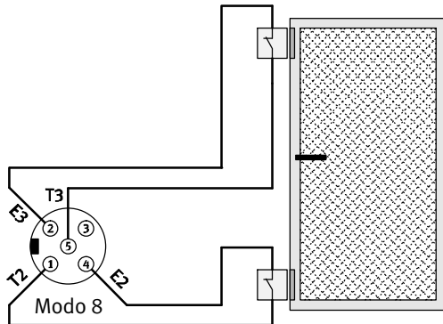
Fig. 1/10: 2 interruptores NO en un par de canales
