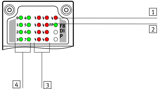
Bild 4/1: LED-Anzeige des Eingangsmoduls CPX-F8DE-P
