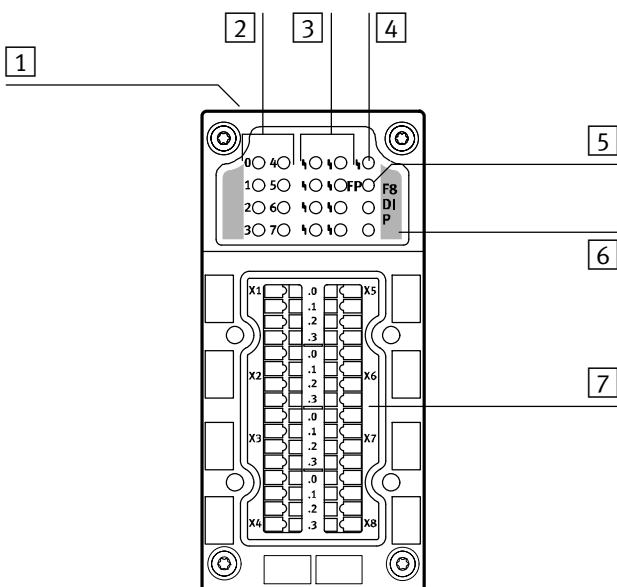
Bild 2/1: Anzeige- und Anschlusselemente CPX-F8DE-P
