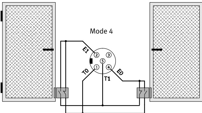
Fig. 1/9 : 2 capteurs de porte de protection à une paire de canaux
