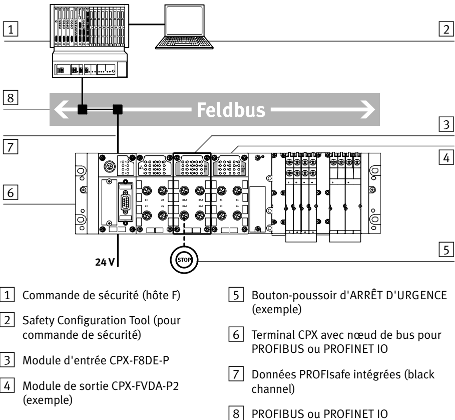
Fig. 1/2 : Communication entre commande de sécurité et modules de sécurité via PROFIsafe
