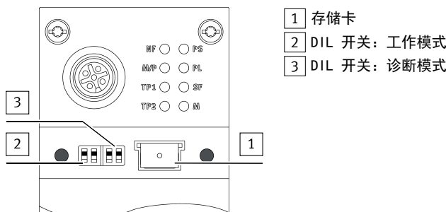
Fig. 2 PROFINET 操作元件
