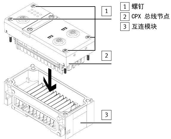
Fig. 3 互连模块中总线节点的安装
