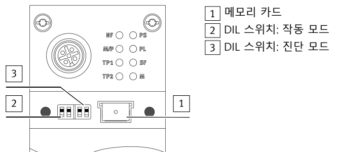
Fig. 2 PROFIBUS용 조작부
