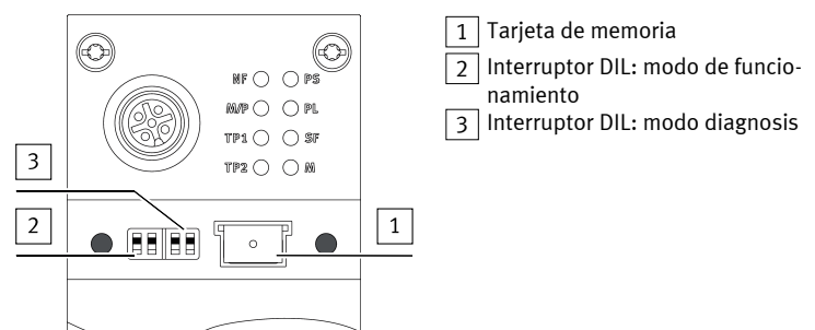
Fig. 2 Elementos de mando para PROFINET
