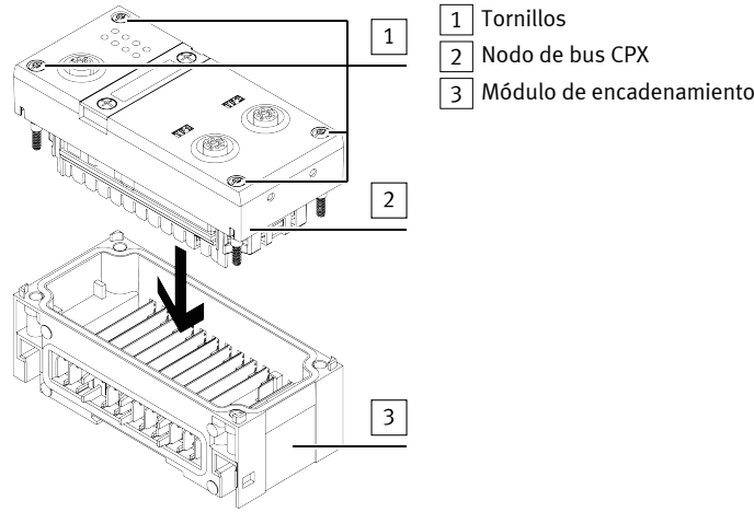
Fig. 3 Montaje del nodo de bus en un módulo de encadenamiento
