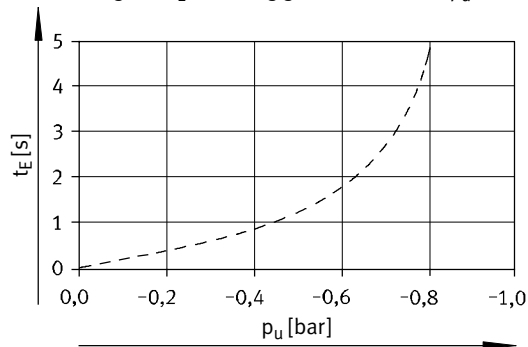
Evakuierungszeit t_E in Abhängigkeit vom Vakuum p_u
