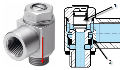
Fig. 23. Snelheidsregelventiel FESTO type GRLZ-1/8-B
